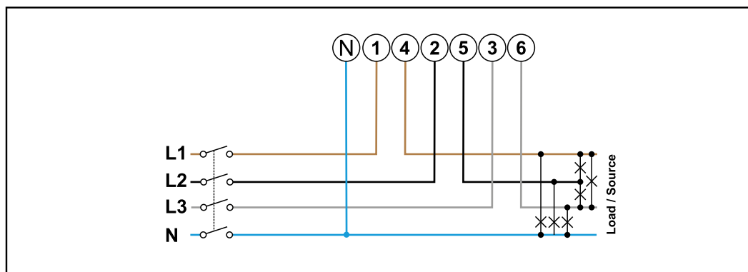
3 fazy, 4 przewody
